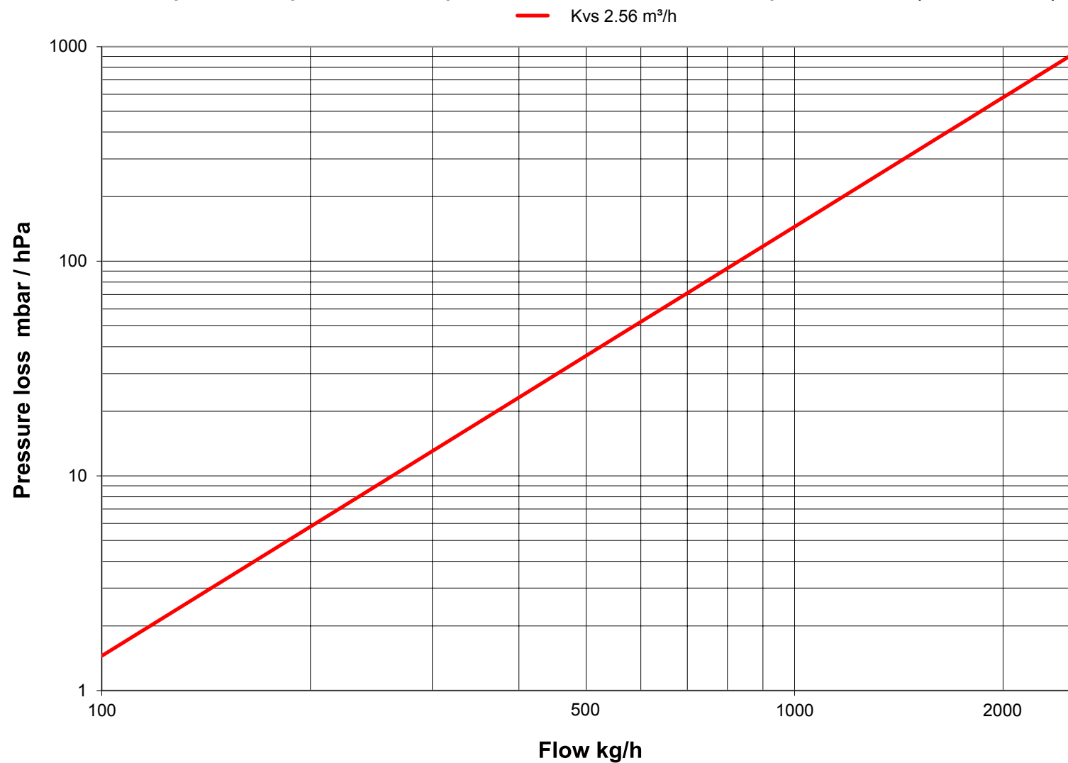
Диаграмма потерь давления термостатических вентилей на обратной линии (EMi02, EMi03)
